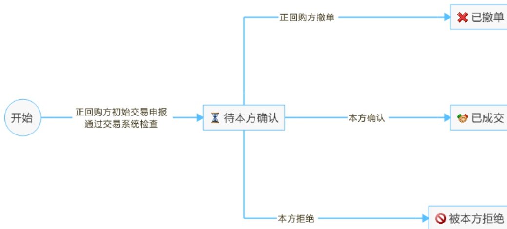
图 5.2-10 逆回购方初始交易申报状态切换图
