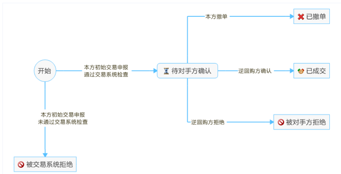
图 5.2-5 正回购方初始交易申报状态切换图
