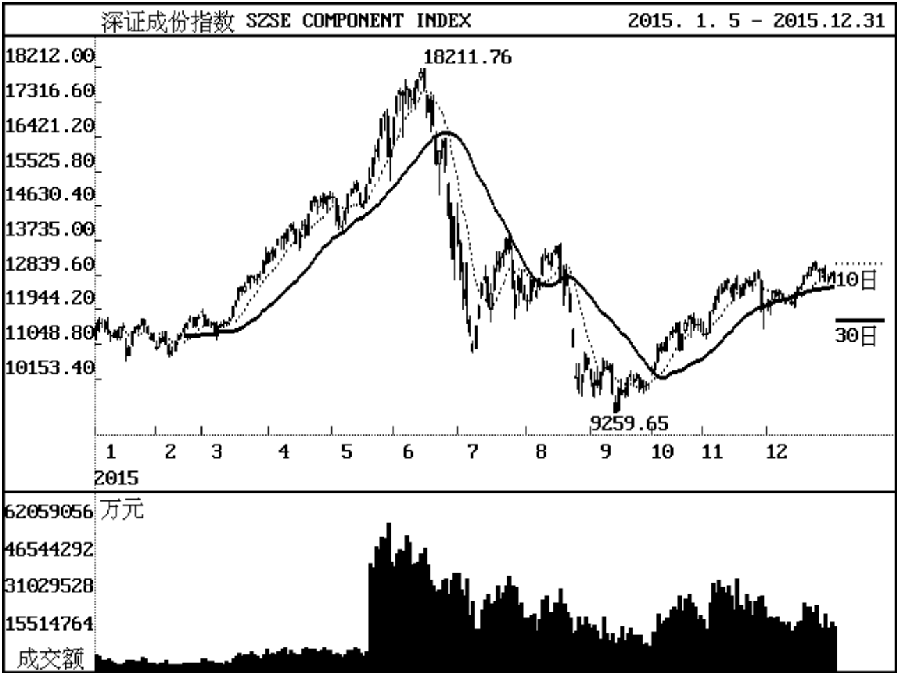
7. 深证成份指数全年走势图(二〇一五年) SZSE COMPONENT INDEX, DAILY MOVEMENT CHART, 2015
